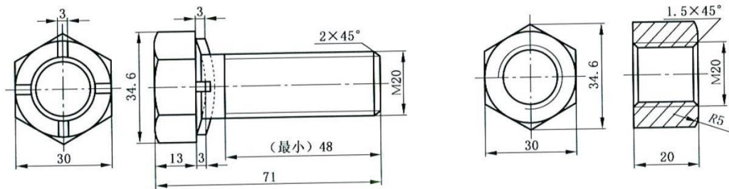
图 A.4 M20×55 带爪螺栓、螺母
