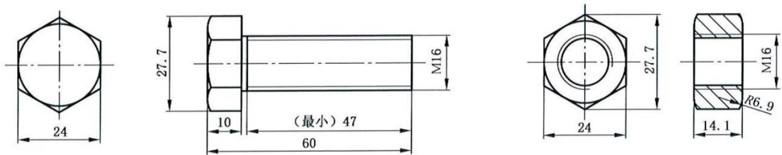
图 A.2 M16×50 螺栓、螺母
