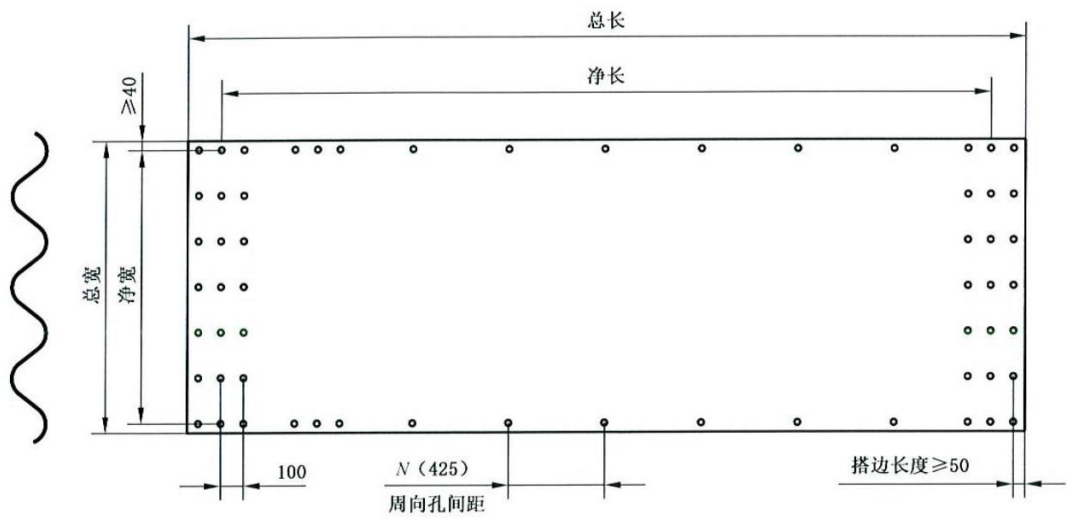
图 11 大波波纹钢板件板型示意图
