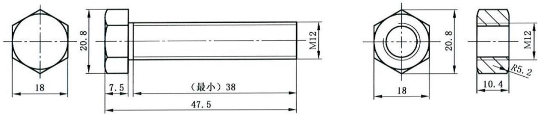
图 A.1 M12×40 螺栓、螺母
