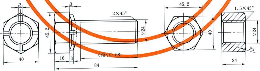
图 A.6 M24×70 带爪螺栓、螺母
