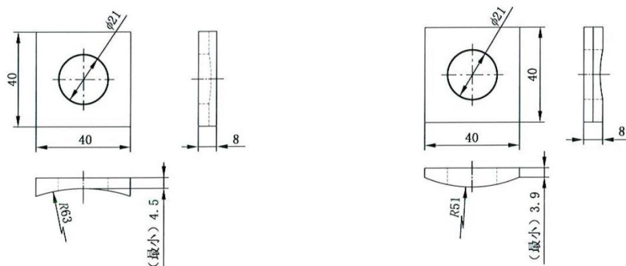
图 B.3 M20 螺栓凹凸垫圈(适用于 200 mm×55 mm、230 mm×64 mm 波形)
